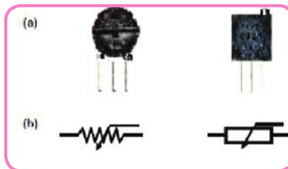
Sumber : Dokumen Kemdikbud Gambar 2.3. Resistor variabel
