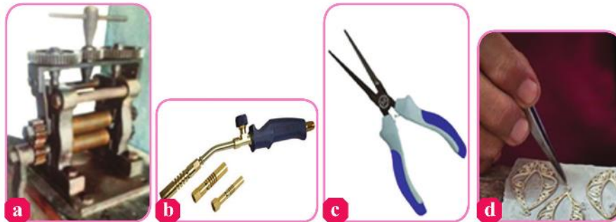
Sumber : Dokumen Kemdikbud Gambar 1.23. Plat kerajinan logam; a. Alat penggiling logam menjadi plat, b. alat patri, c. tang lancip, d. penjepit.
